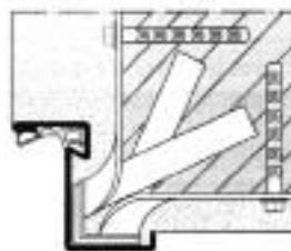
Saroktok dűbeles rögzítéssel kombinálva
