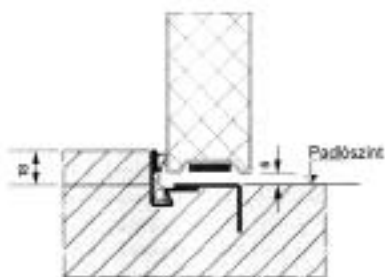
TAE-A T30 alsó ütközővel
